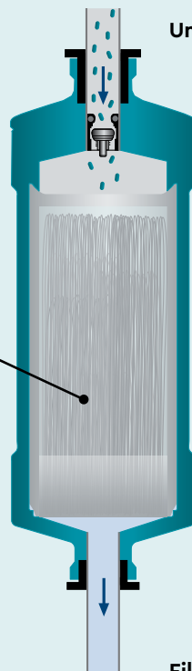
BWT BESTCARE MINI FILTER CARTRIDGE
